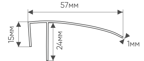
F-профиль 55*1 артикул: W005/1
