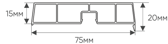
Прямой 75мм артикул: W601
