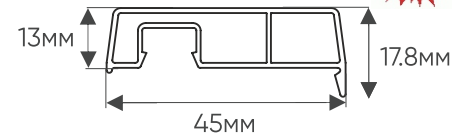
Прямой 45мм артикул: W607
