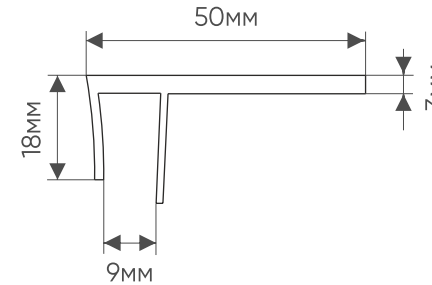
F-профиль 50*3 артикул: W005
